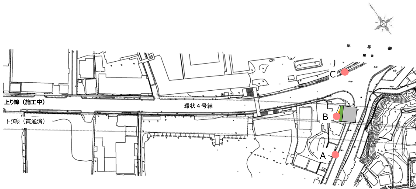
【シールドマシン位置図（1月21日時点）】
